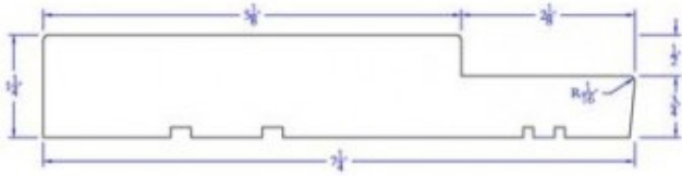
Exterior Kerfed Jamb
