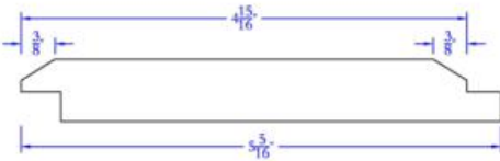
Fingerjoint - WC 137
