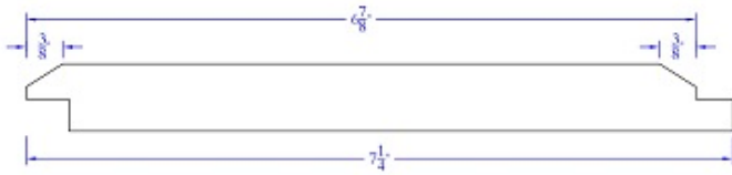
Fingerjoint - WC 137
